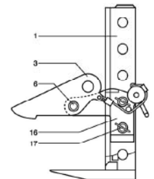
Onderdelen voor IPPE veiligheids-hijsklemmen:
